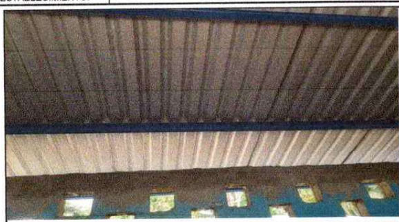
foto 1: Sustitución de lámina, por lámina troquelada aluzinc calibre 26 AULAS 8,9 Y PATIO
